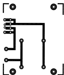
CIRCUIT DECODEUR
