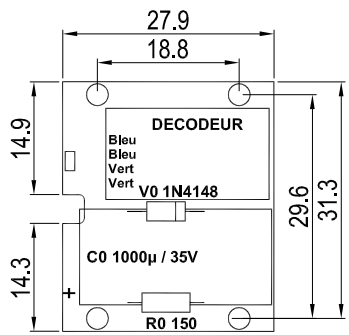
CIRCUIT DECODEUR
