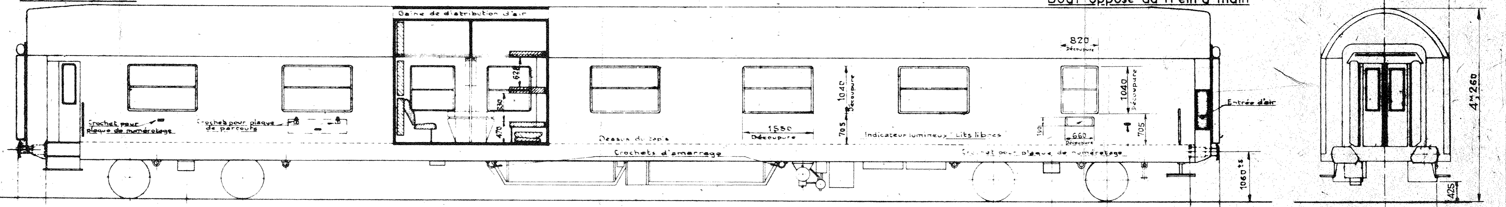
Bout frein à main VUE COTE COULOIR Bout opposé au frein à main
